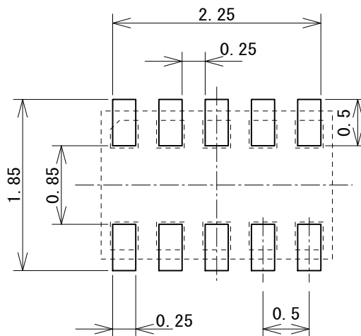
●参考メタルマスクデザイン/ Reference Metal Mask Design
